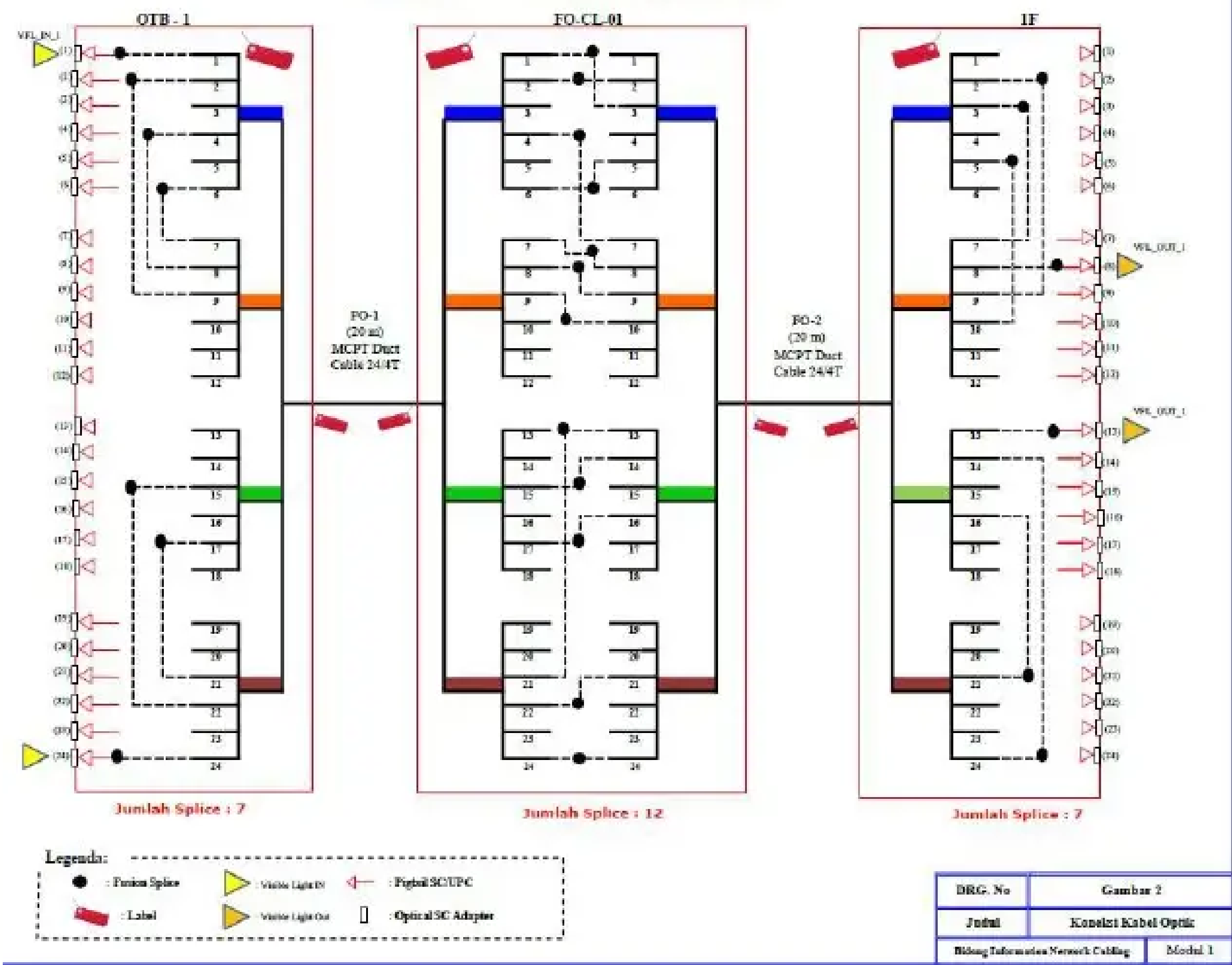
Gambar 1 Skematik Modul 1
